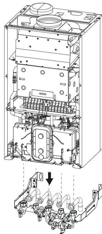
schéma 5 - Remplacement avec Kit barrette 3319211 (URBIA) 3319208 (SERELIA) sans cadre écarteur
