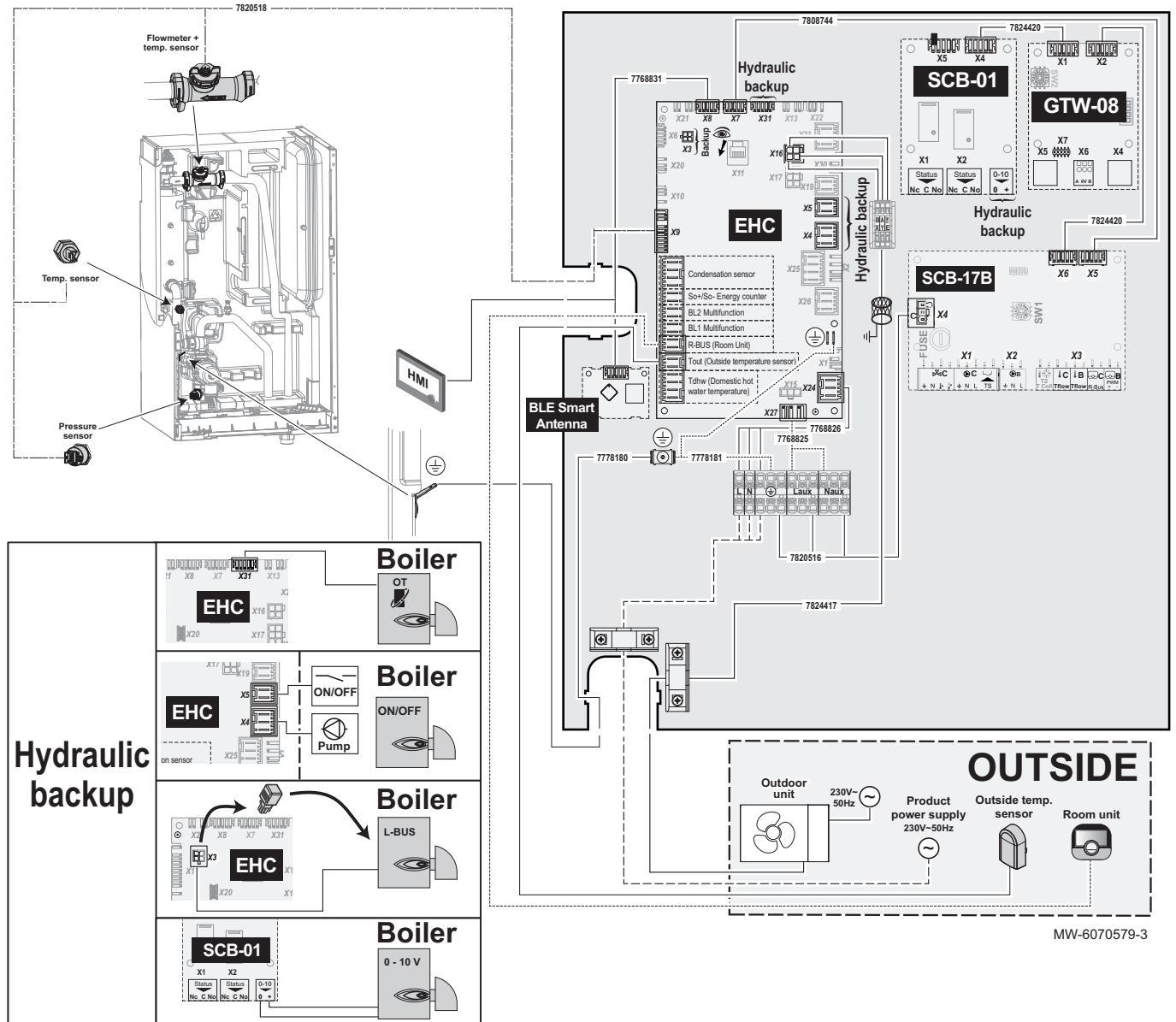
Fig.9 MIV-M /H avec appoint hydraulique
