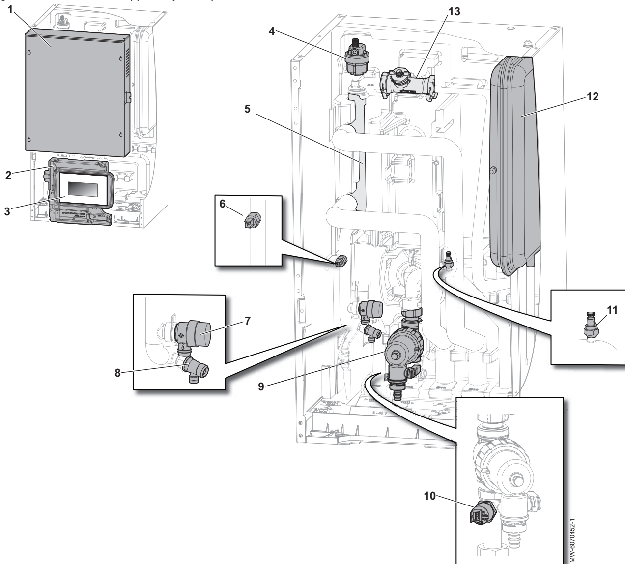
Fig.13 MIV-M /H avec appoint hydraulique
