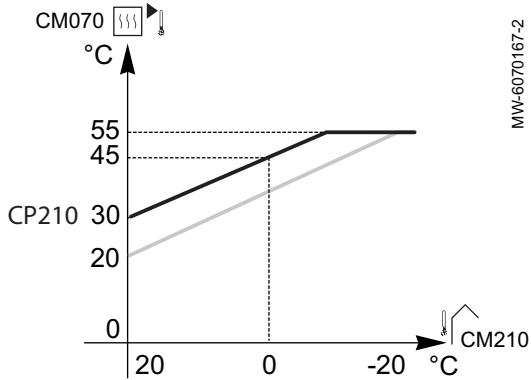
Fig.79 Courbe de chauffe avec pied de courbe
