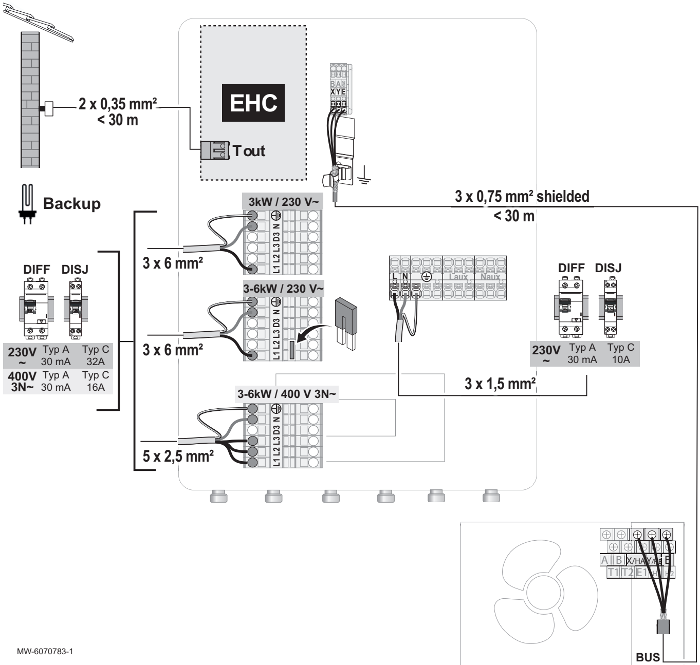
Fig.40 Groupes extérieurs MONO AWHP3R et MIV-M /E avec résistance électrique 3-6 kW
