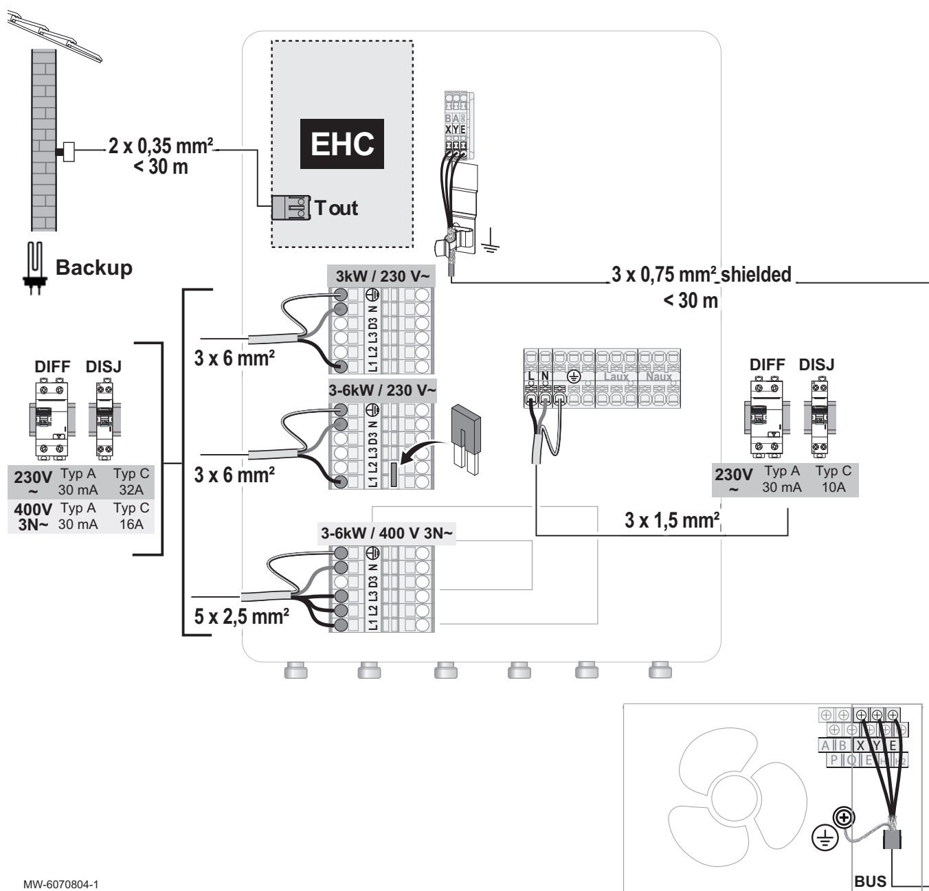
Fig.41 Groupes extérieurs MONO AWHP2R et MIV-M /E avec résistance électrique 3-6 kW
