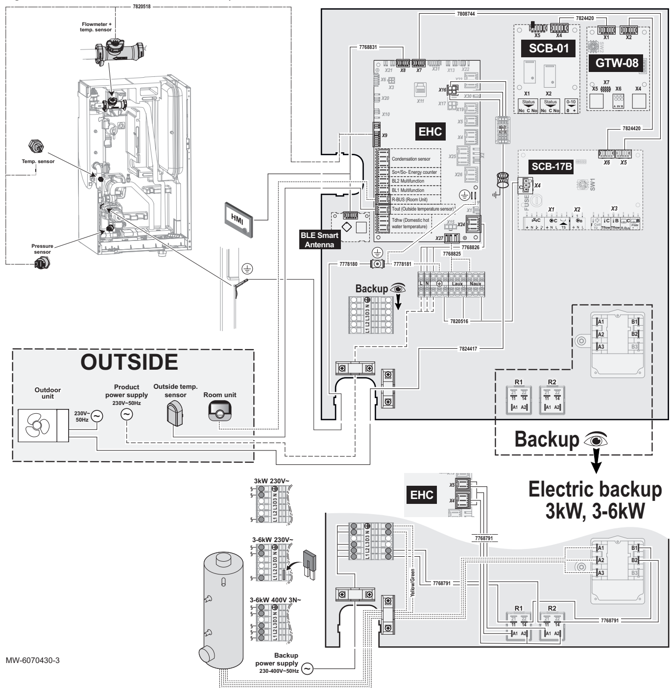
Fig.8 MIV-M /E avec résistance électrique
