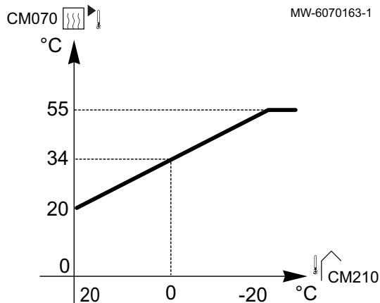
Fig.78 Courbe de chauffe sans pied de courbe
