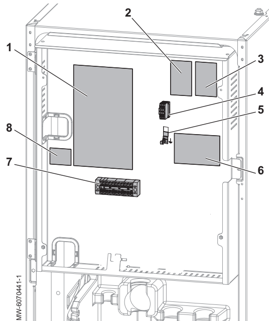
Fig.15 MIV-M /H avec appoint hydraulique
