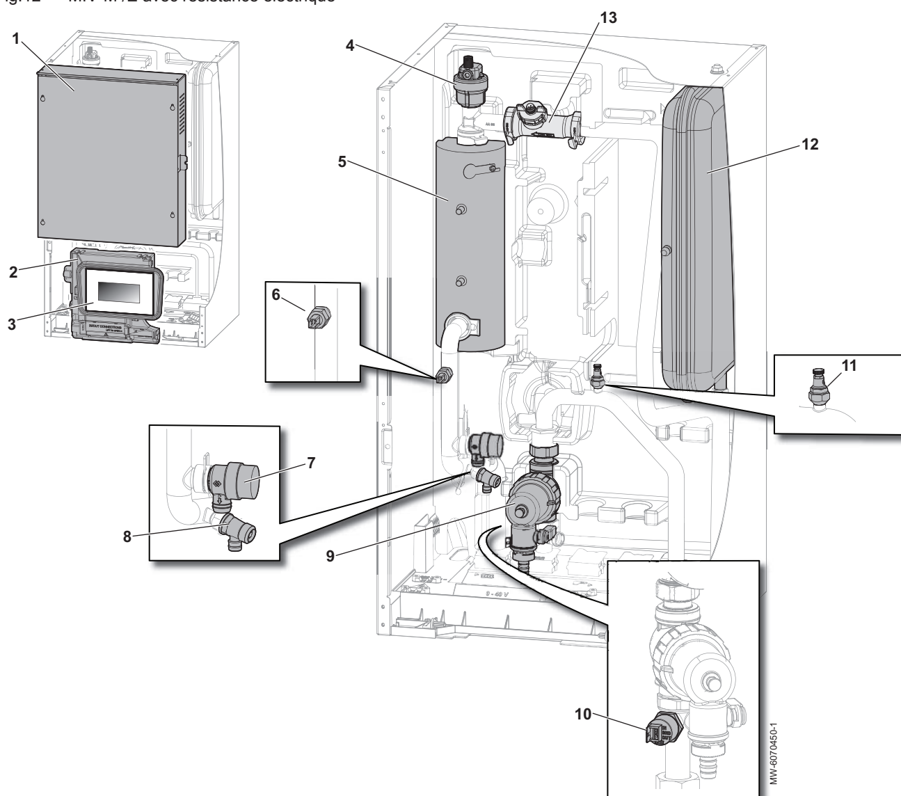
Fig.12 MIV-M /E avec résistance électrique
