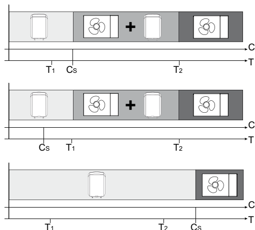
Fig.71 Influence des températures extérieures et de bivalence.
