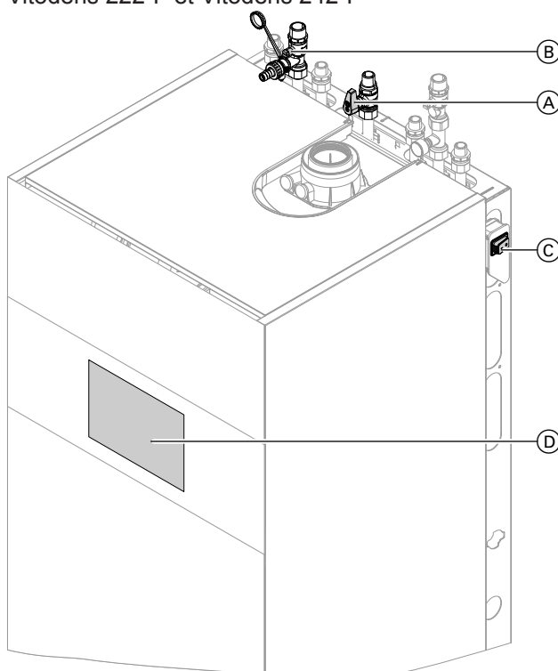
Fig. 15 Exemple avec les raccordements vers le haut
