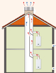
Conduit Shunt ou Alsace Voir DTU 241 P2
