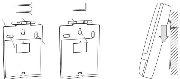
3. Utiliser les trous pour fixer le support sur le mur
