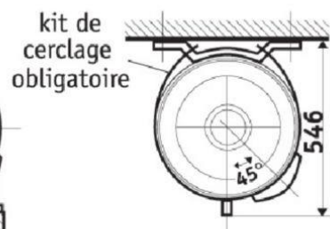
Montage au plafond
