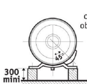
Montage au sol
