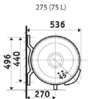
Montage au mur
